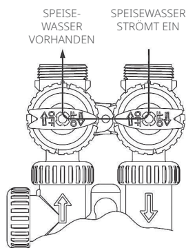
BYPASS-BETRIEB
