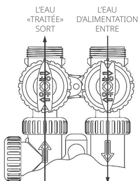
FONCTIONNEMENT NORMAL
