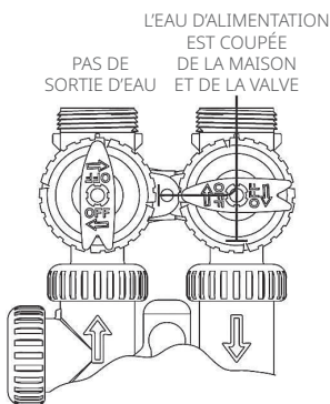
MODE D'ARRÊT
