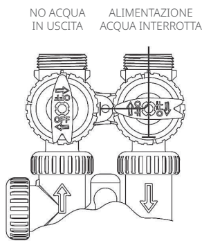
MODO SPEGNIMENTO
